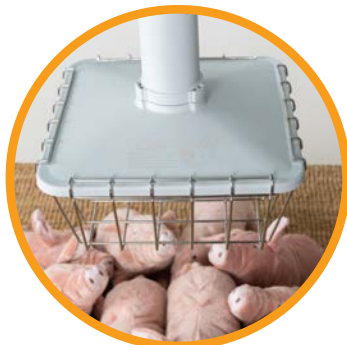
SOLAR 225 Lampe chauffante 225W
